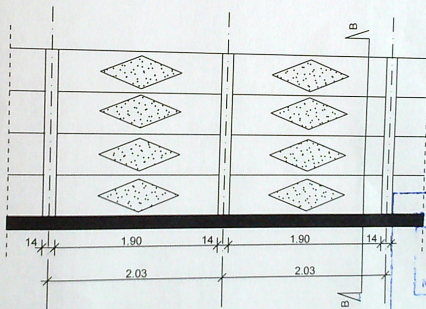
VEDERE LATURA EST SC. 1:50 imprejmuire prefabricate
